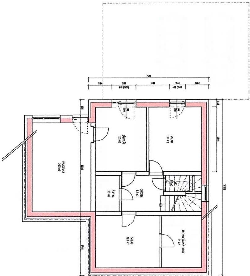
PŮDORYS 1.PP
