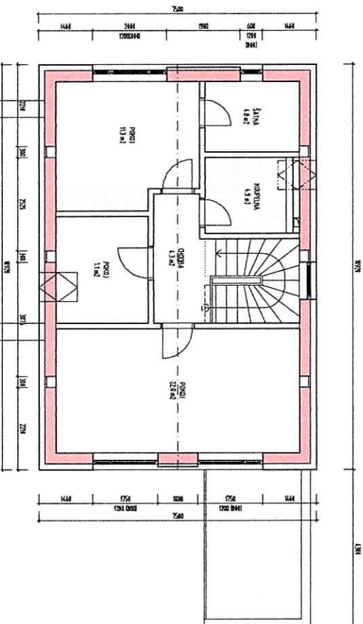
PŮDORYS PODKROVÍ
